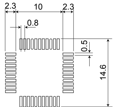
裏面 QFP44ピン/0.8
