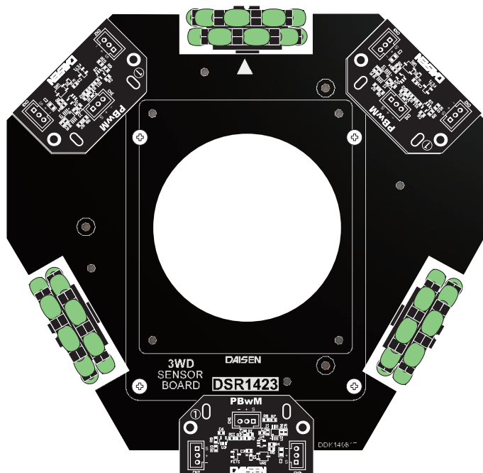
3 輪用センサーボード
