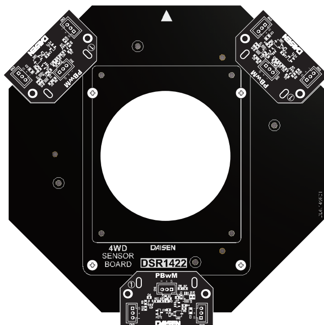
4 輪用センサーボード
