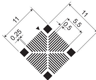
裏面 QFP48P/0.5
